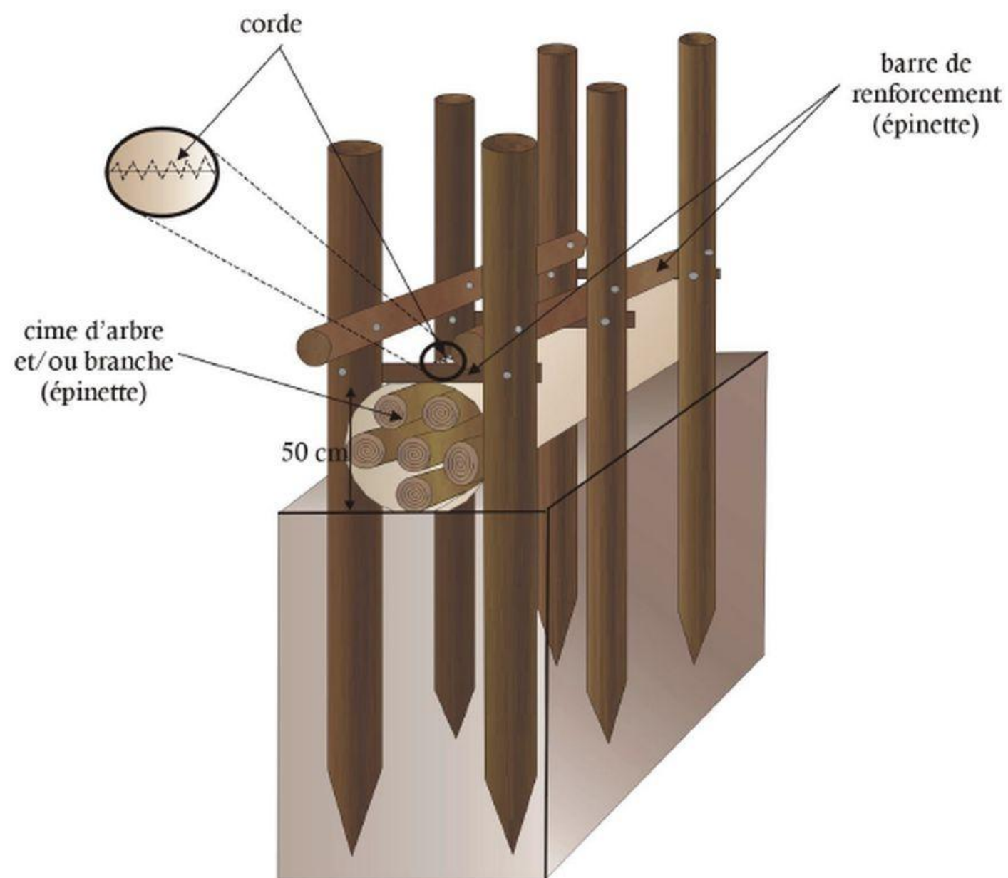
Figure 11. Pile fondation et système de renforcement.
