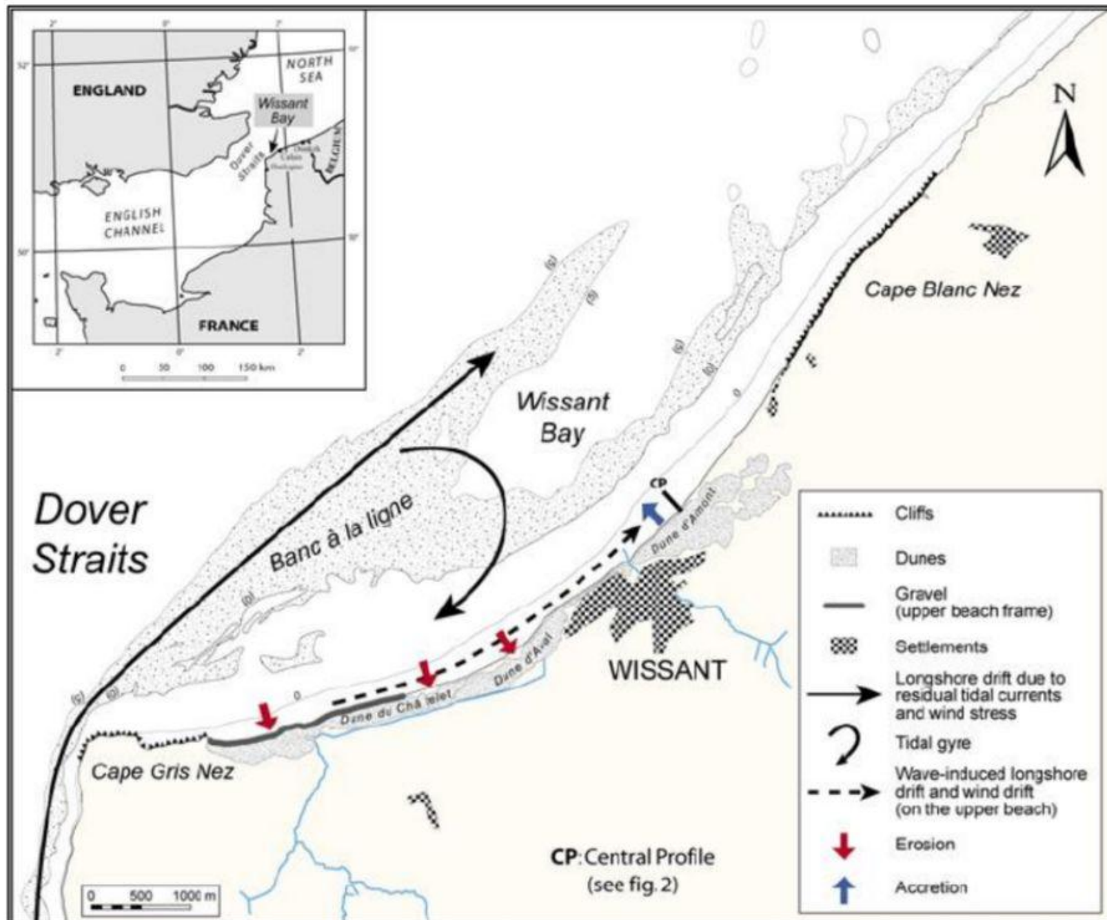
Figure 29: Morphologie et dynamique sédimentaire en baie de Wissant (Sedraty & Anthony, 2006 ; [A10])
