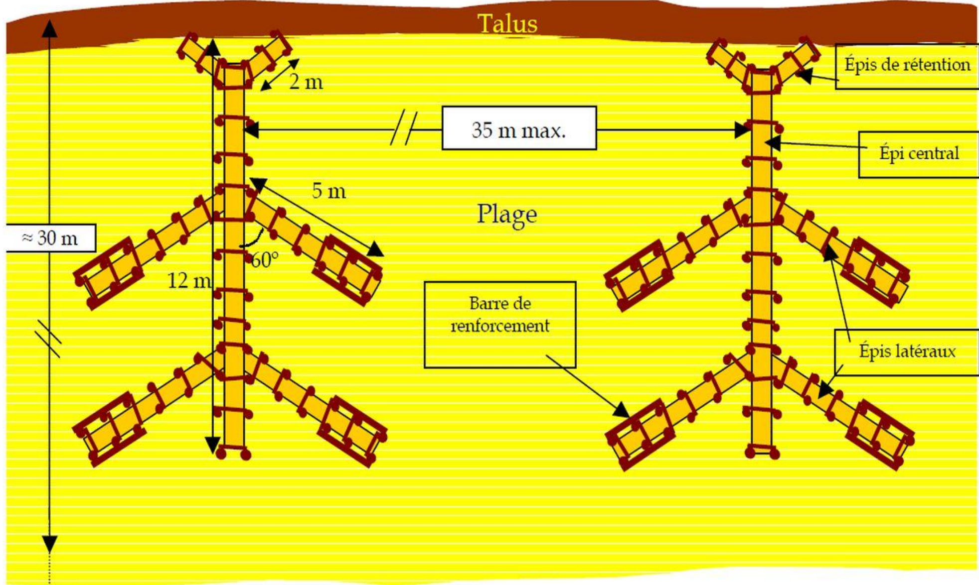
Figure 6 - Positionnement optimal des SEMS sur la plage
