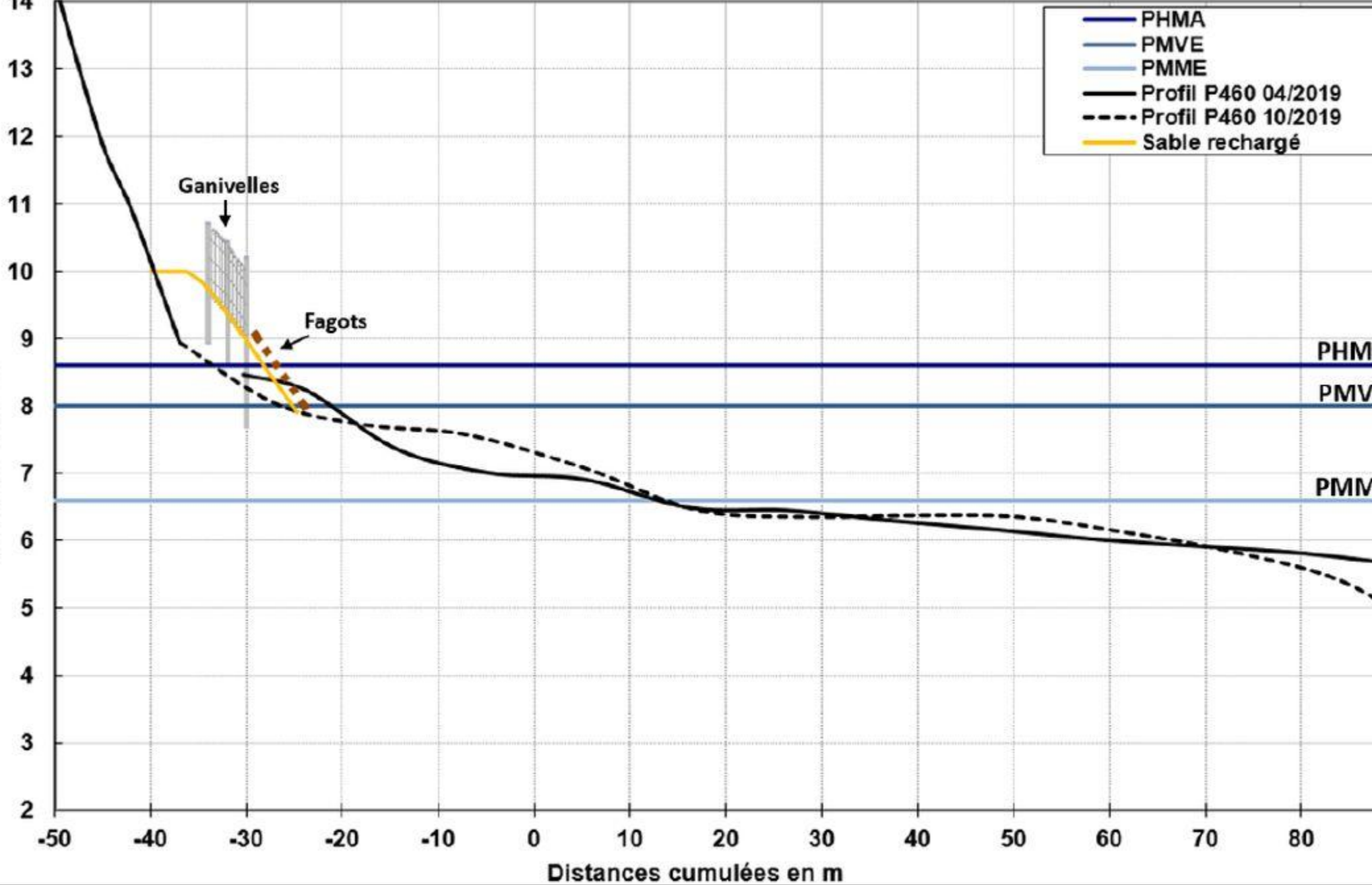
Figure 80 : Coupe-type des aménagements envisagés en Priorité 2 sur le secteur Dune d'Am... (montée de sable, fagots et ganivelles)
